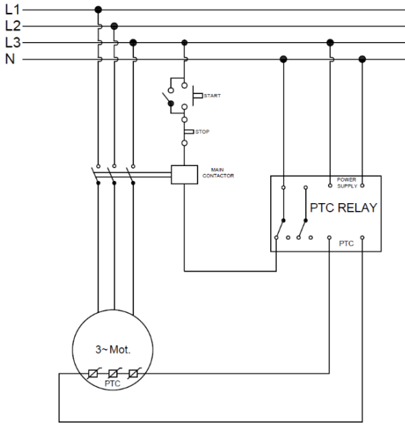
Termistör Bağlantısı
